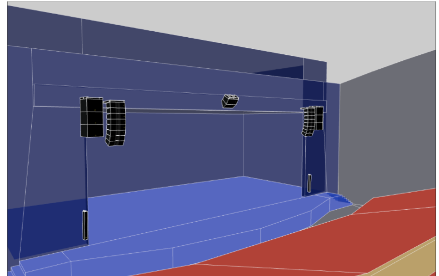
Vue latérale du système.
